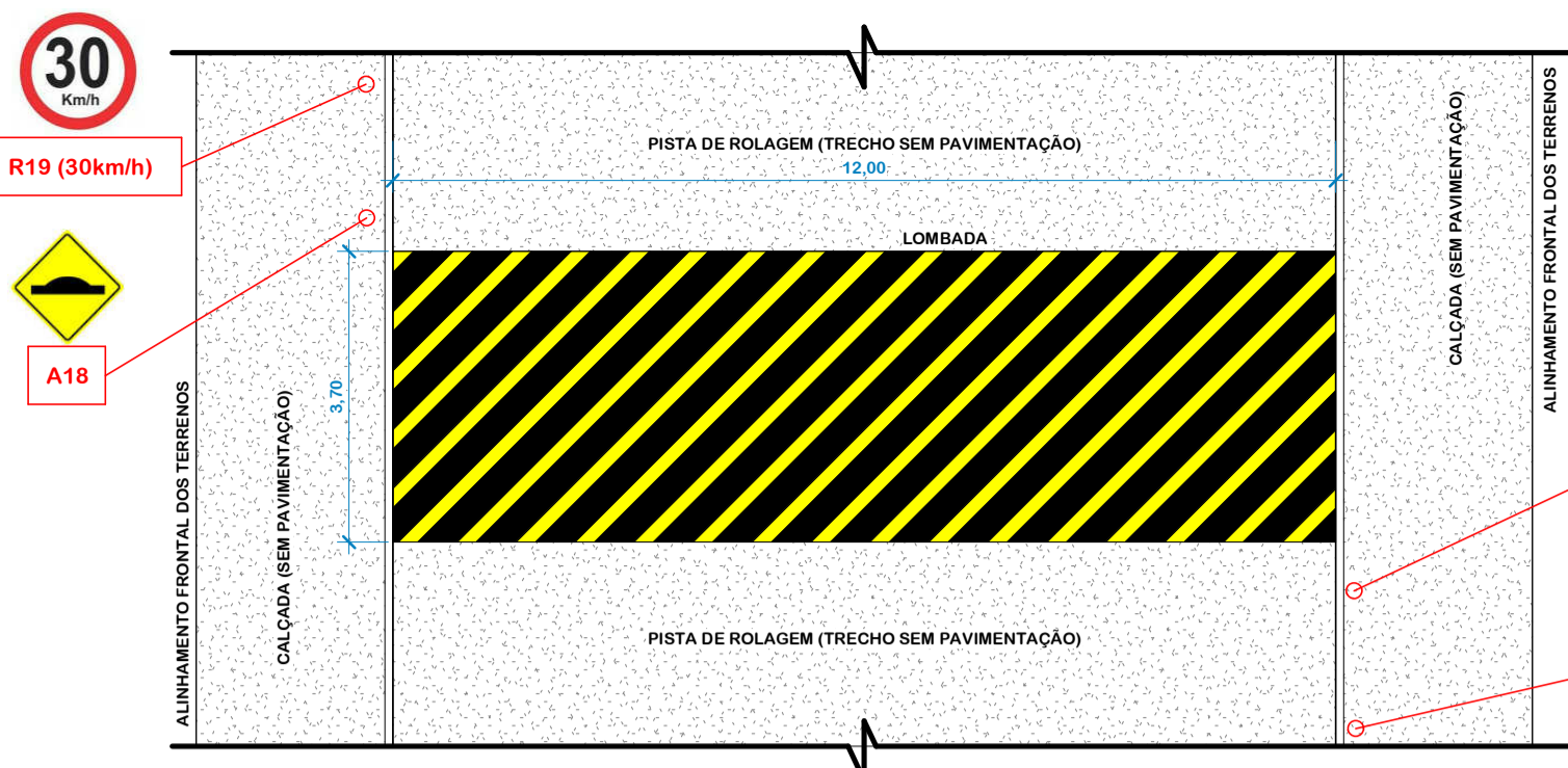
GABARITO DAS LOMBADAS EM PISTA SEM PAVIMENTAÇÃO Esc.: 1 : 100
