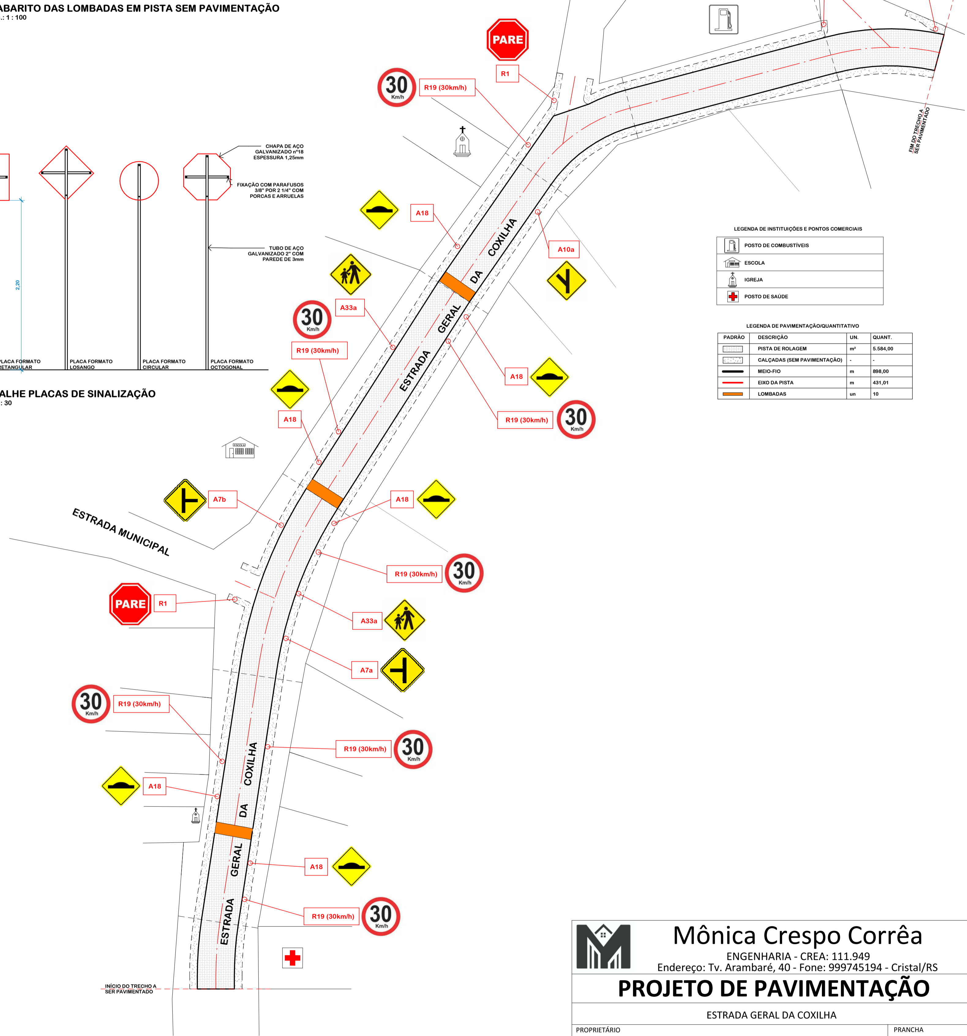
LOCAÇÃO DAS PLACAS DE SINALIZAÇÃO Esc.: 1 : 750
