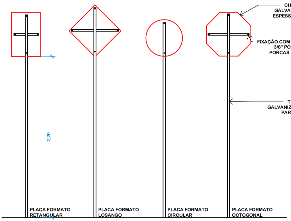
DETALHE PLACAS DE SINALIZAÇÃO Esc.: 1 : 30
